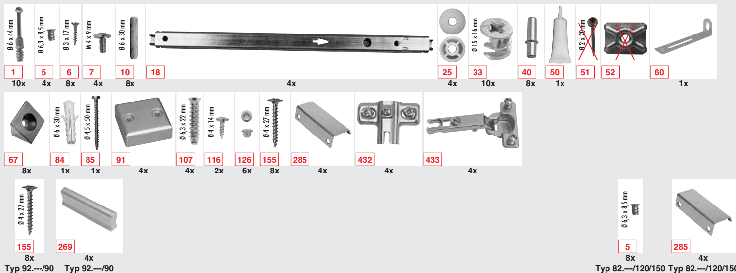
Typ 92.---/90 B 71 cm • H 75 cm • T 35 cm
