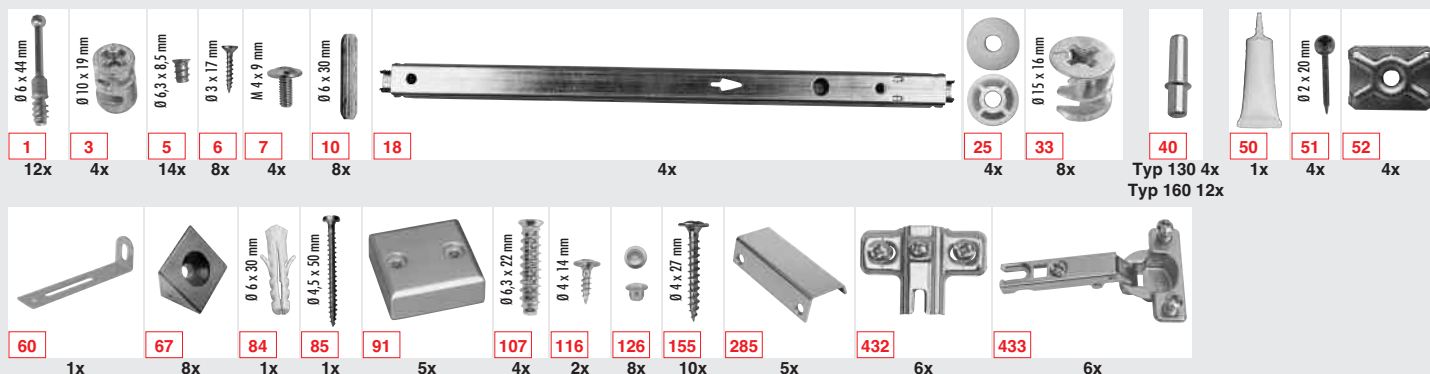
Typ 82.---/130 B 106 cm • H 75 cm • T 35 cm
